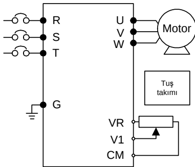
Kablolama
